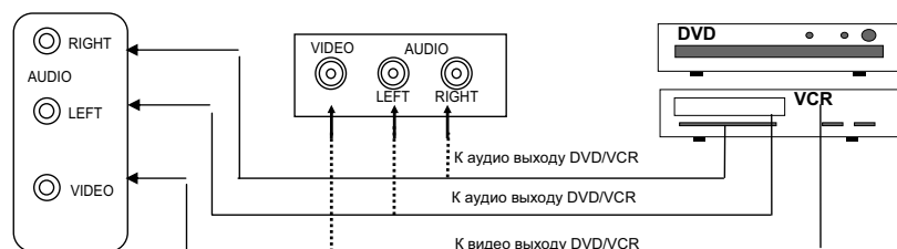
Схема 2. Подключение внешних устройств (DVD, VCR,...) через AV In (на боковой или передней панели)
