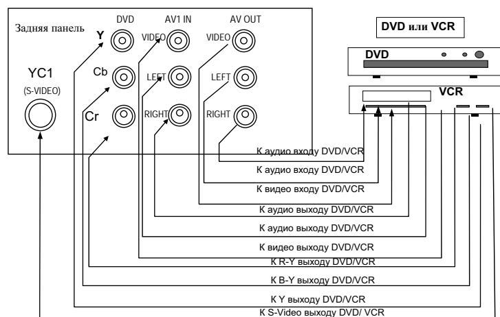
Схема 1. Подключение внешних устройств (DVD, VCR,...) через AV1 In, AV Out, DVD (YCbCr), YC1 (S-Video) (на задней панели)
